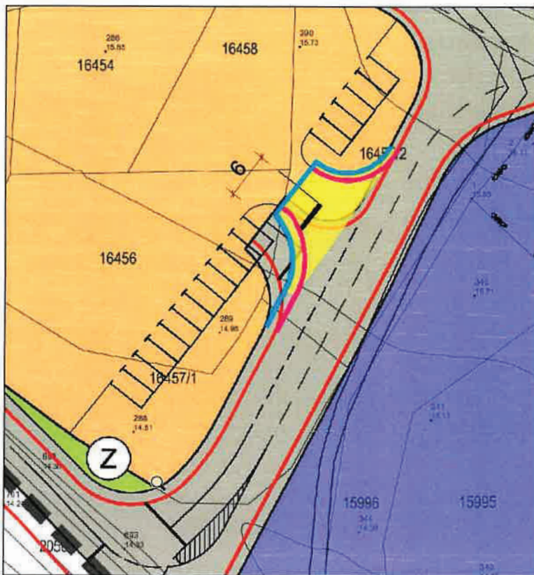
Slika 1. Prijedlog izmještanja kolnog priključka
