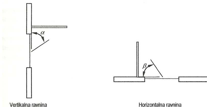
Slika 1.5 Prozorsko zasjenjenje: a) vertikalna ravnina, b) horizontalna ravnina
