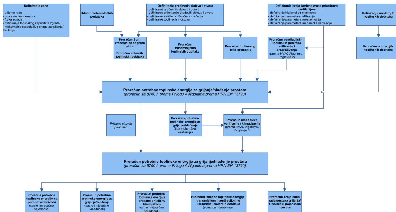
Dijagram toka proračuna potrebne energije za grijanje, hlađenje prostora i mehaničku ventilaciju/klimatizaciju
