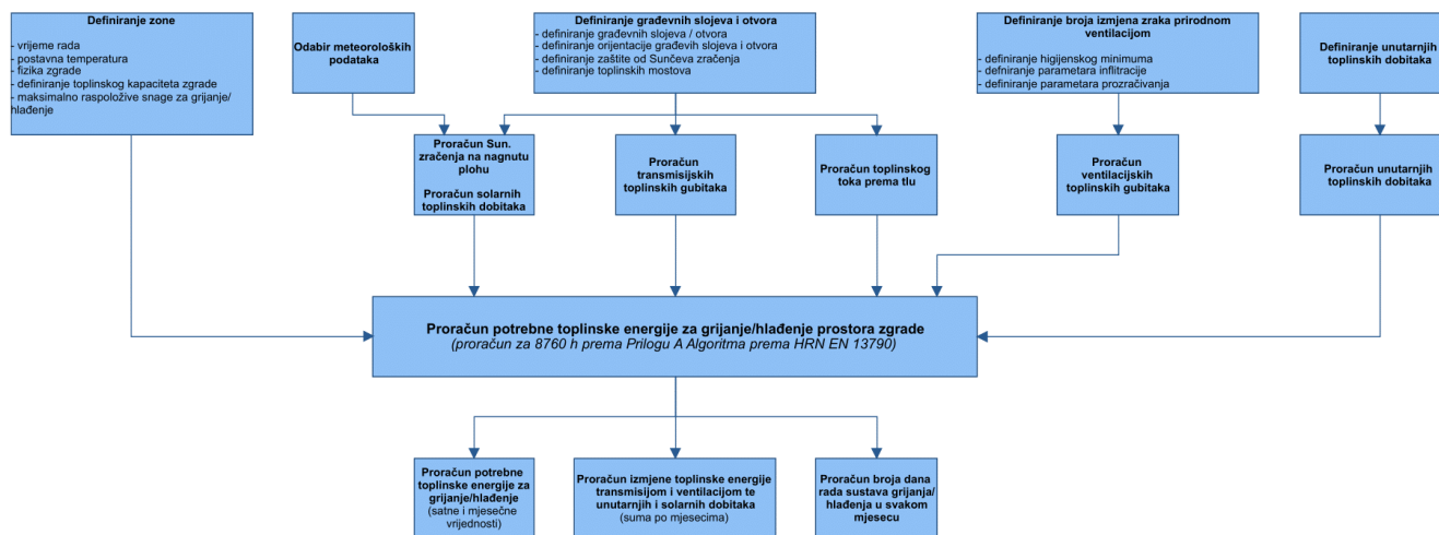
Dijagram toka proračuna potrebne energije za grijanje i hlađenje prostora
