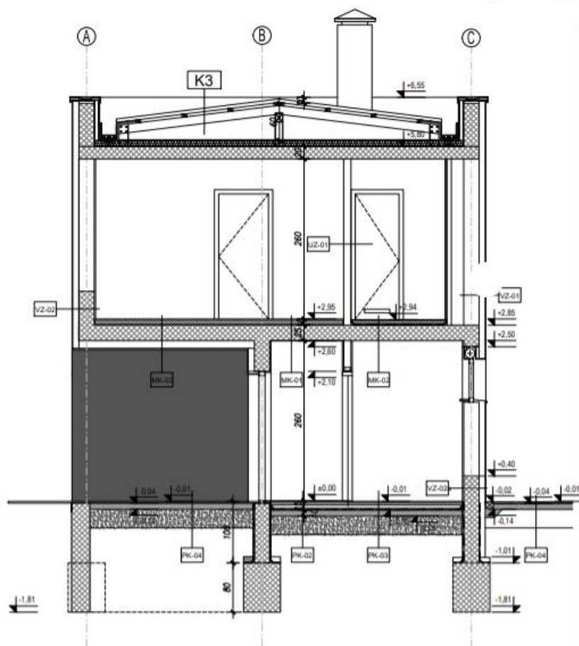
PRESJEK A-A
