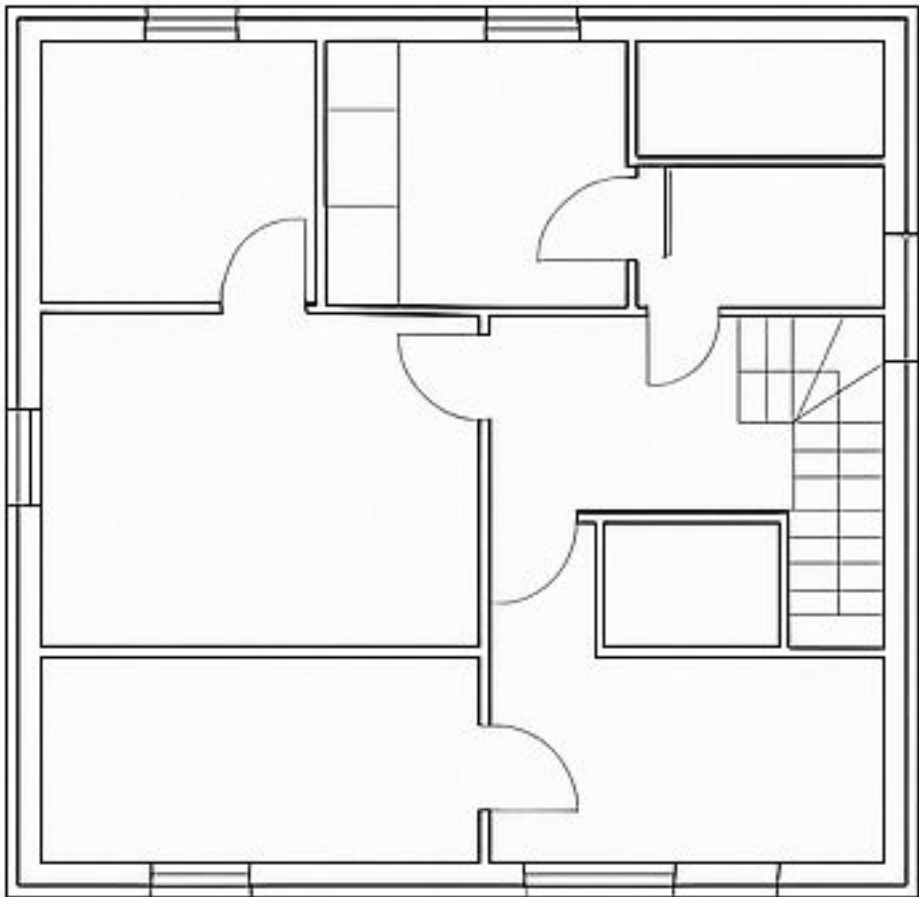
PRIZEMLJE
