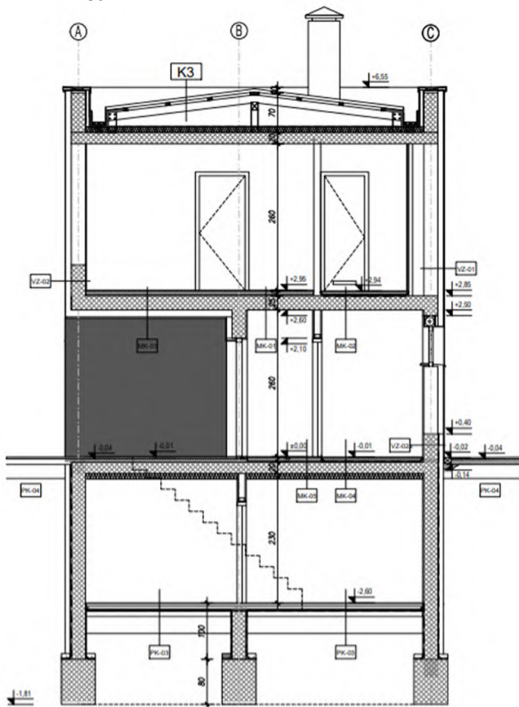
PRESJEK A-A
