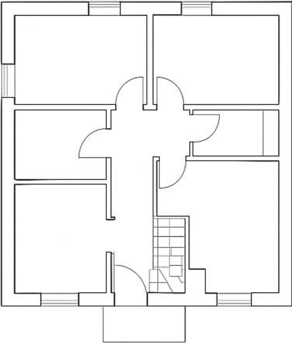
PRIZEMLJE
