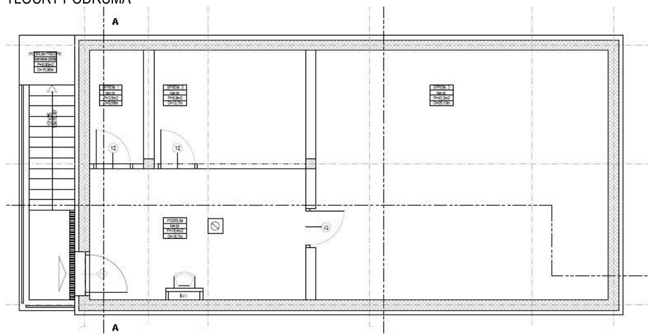
TLOCRT PODRUMA
