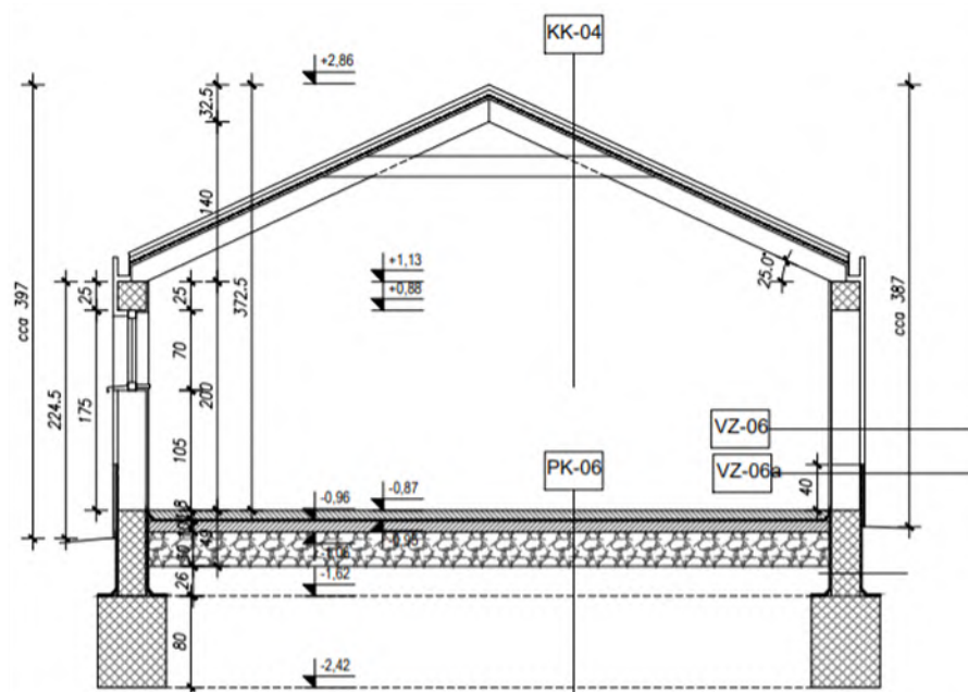
PRESJEK A-A
